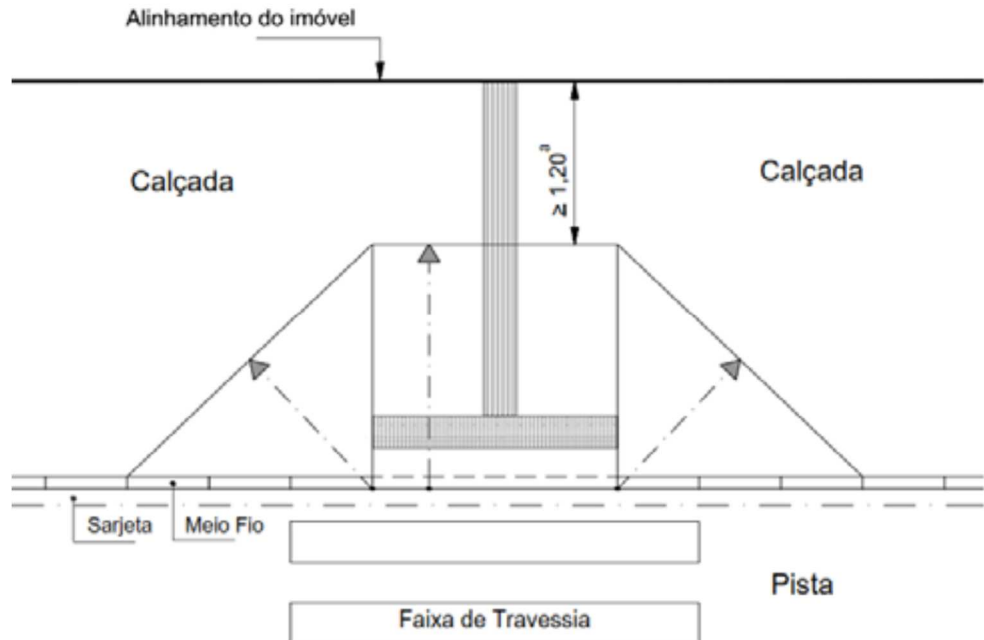
Imagem 01 – Modelo de rampa para Calçadas com 3,00 metros ou mais
